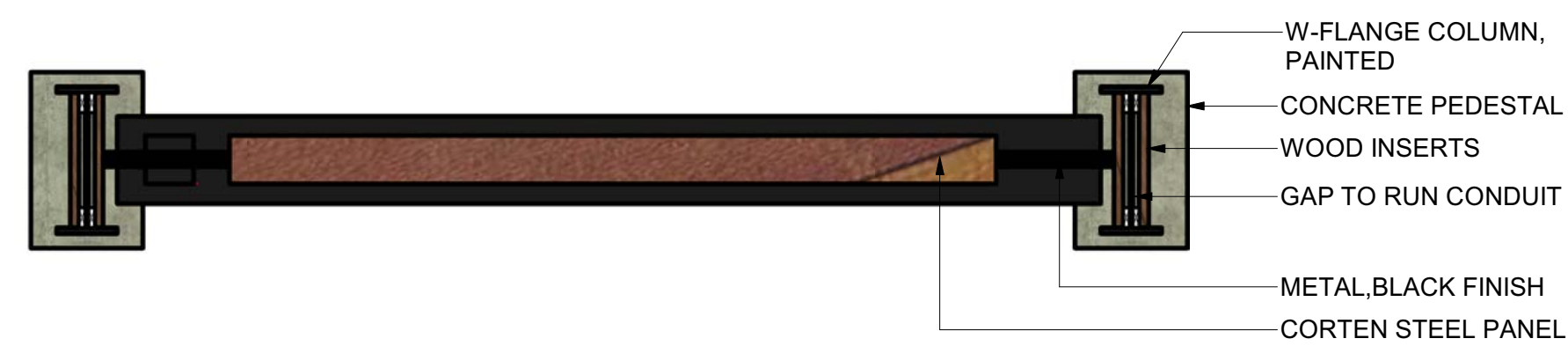
PYLON- PLAN SCALE: 1/2" = 1'-0"
