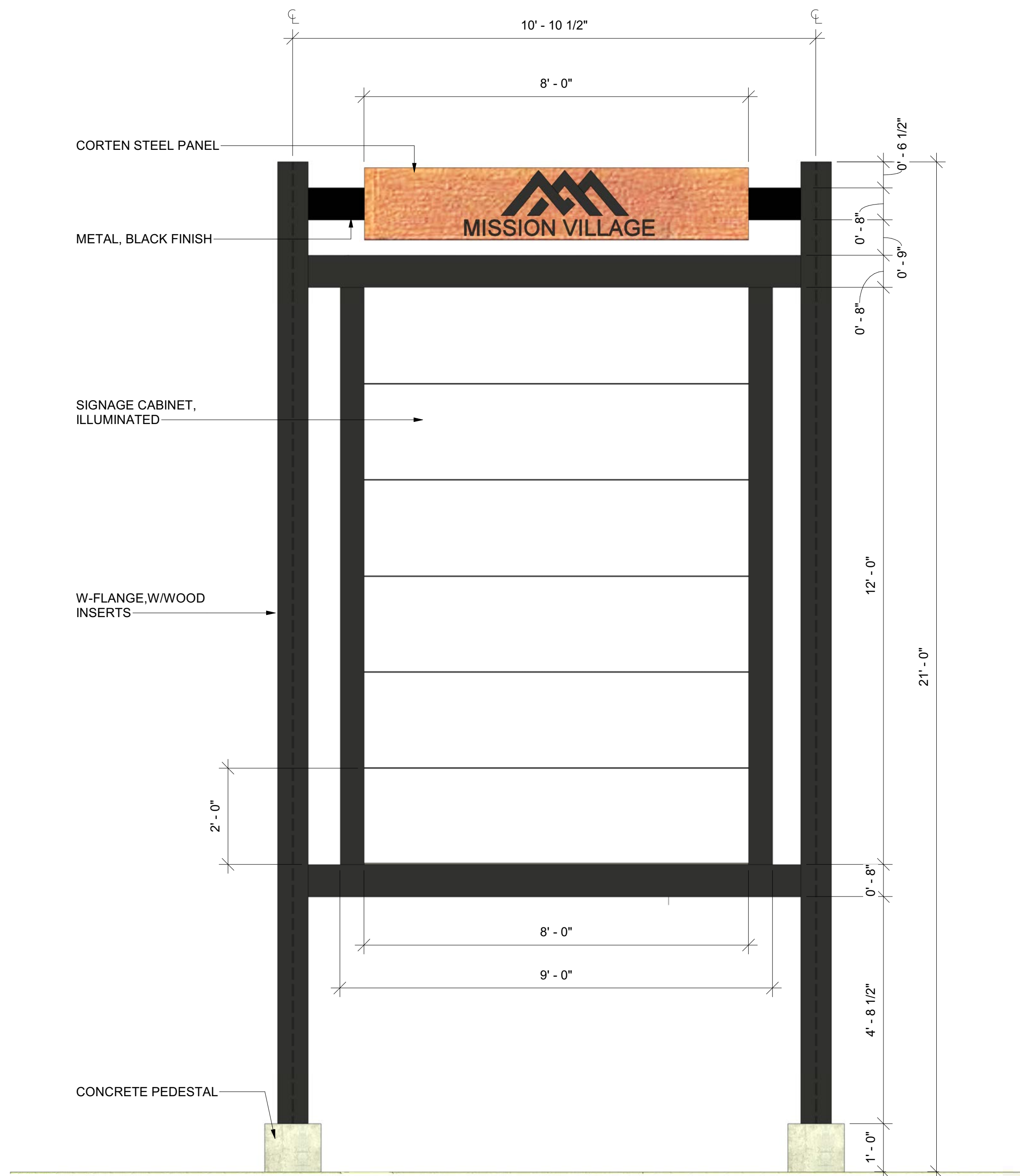
PYLON SIGN SCALE: 1/2" = 1'-0"
